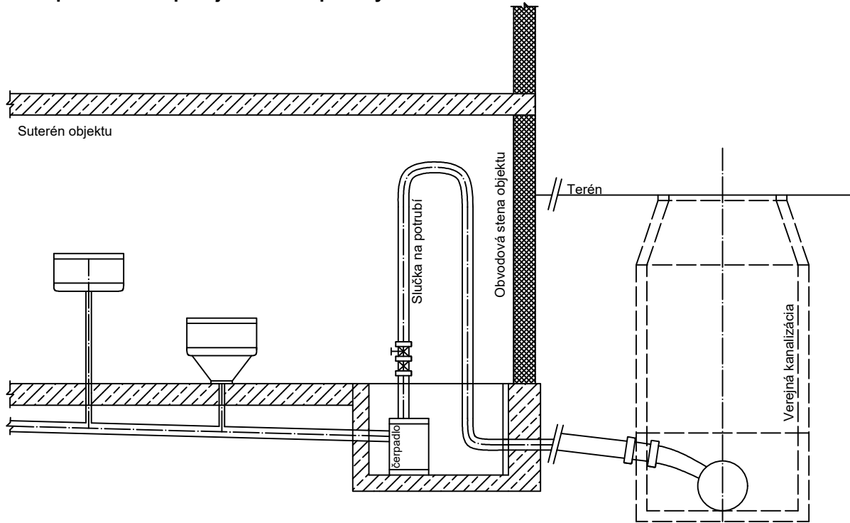
Schéma ochrany proti spätnému vzdutiú pomocou čerpacej stanice odpadových vôd
