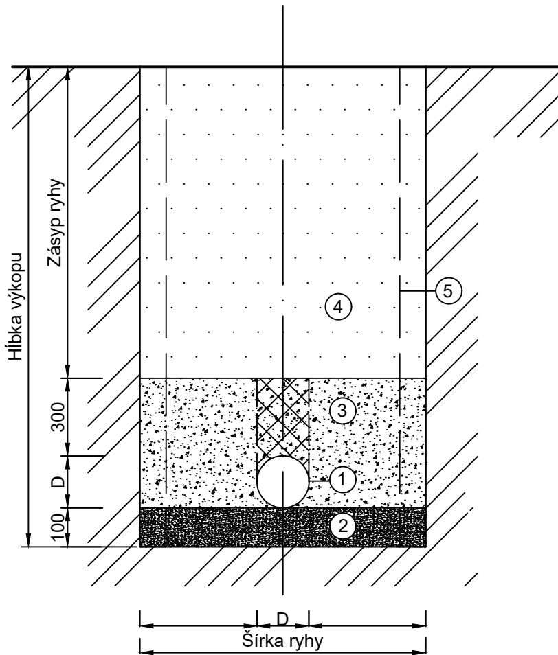
Vzorové uloženie potrubia vodovodnej prípojky
