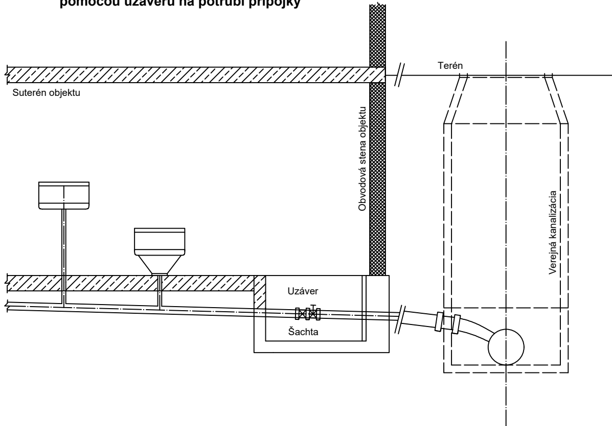
Schéma ochrany proti spätnému vzdutiú pomocou uzáveru na potrubí prípojky
