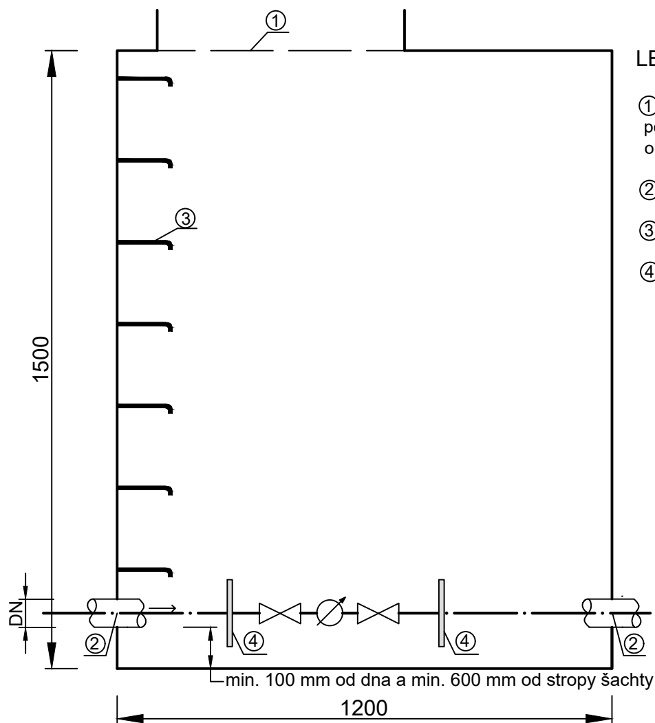
Schéma vodomernej šachty pre vodovodnú prípojku DN 25, DN 32, DN 40, DN 50 s umiestnením dvoch meradiel
